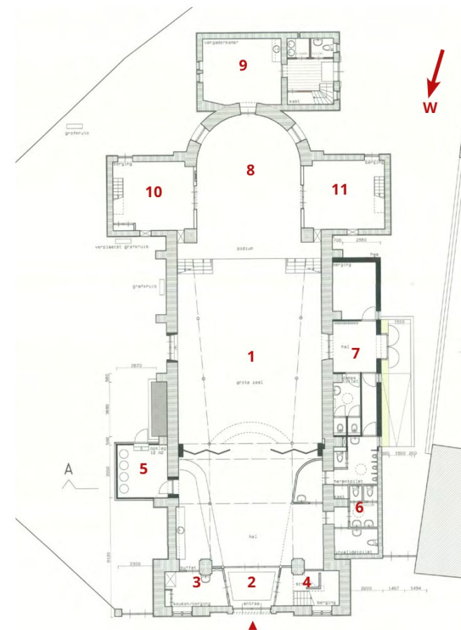
Afbeelding 27 Plattegrond Sint-Agneskerk
