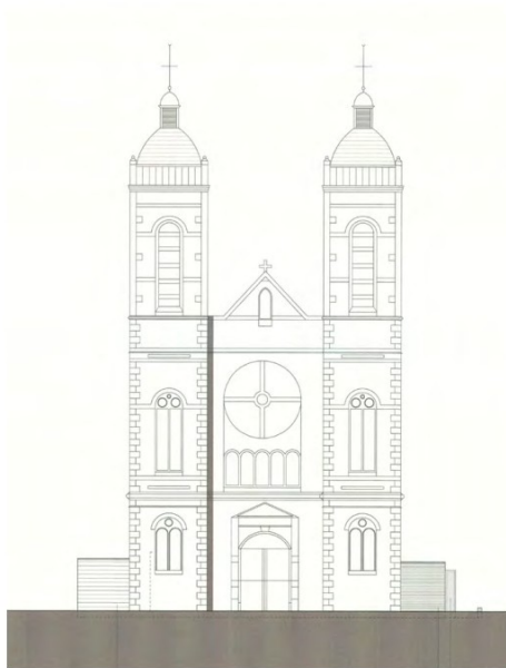
Afbeelding 28 Voorgevel (west)
