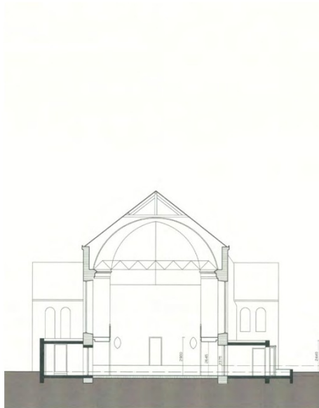
Afbeelding 30 Verticale doorsnede
